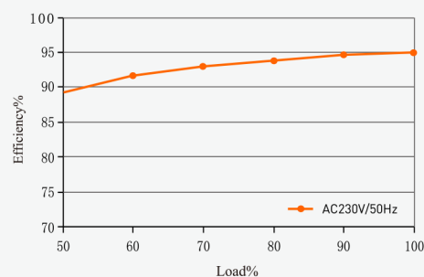
wydajność vs obciążenie / efficiency vs load
